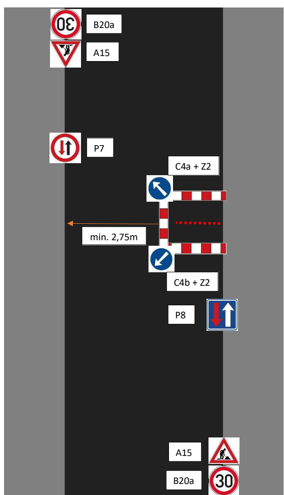
Dopravní značení - překop komunikace po půlkách
