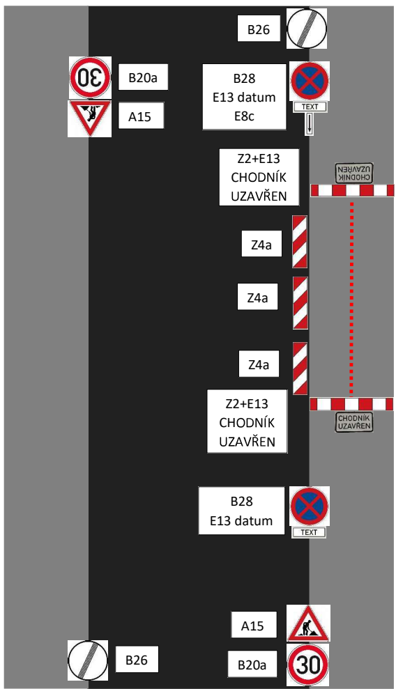
Dopravní značení - výkop v chodníku
